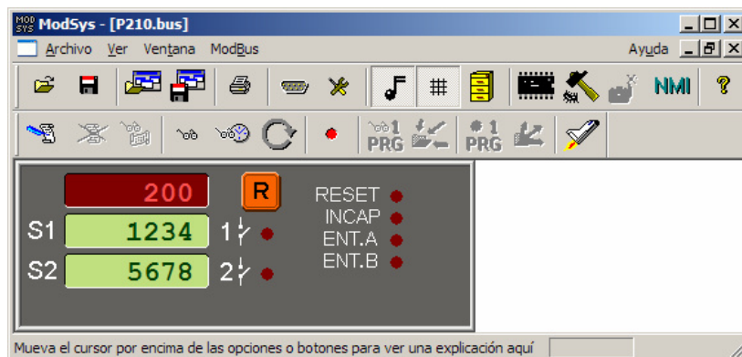
Pantalla de ModSysVR™ monitorizando un P210
